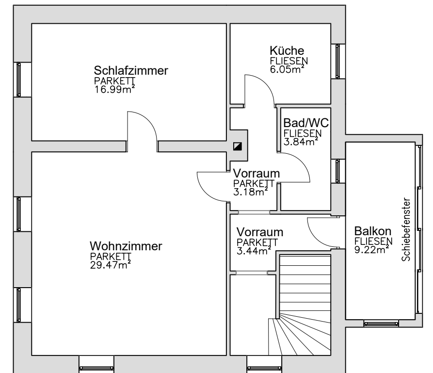
GRUNDRISS 2. OG
