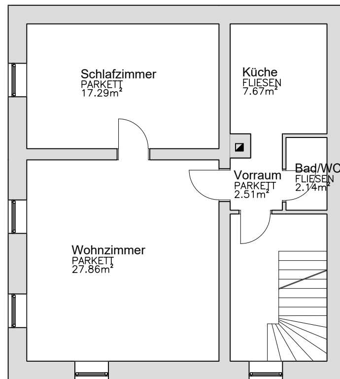
GRUNDRISS 1. OG
