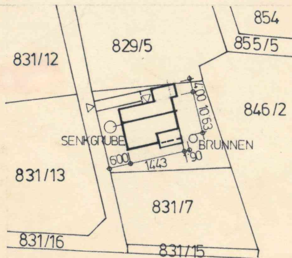
LAGEPLAN 1:1000
